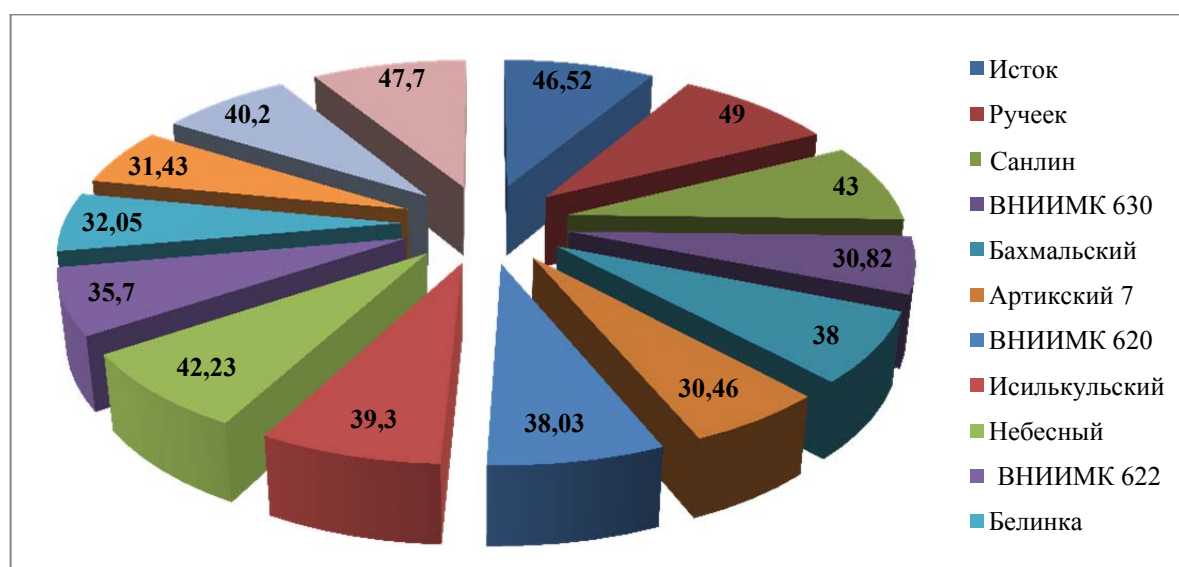
Рис. 2. Содержание жирного масла в льна семенах, %
