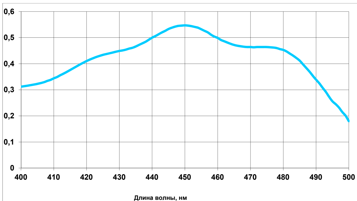
Рис. 1. Спектр поглощения экстракта из плодов рябины (1:25) (ацетоновый раствор)
